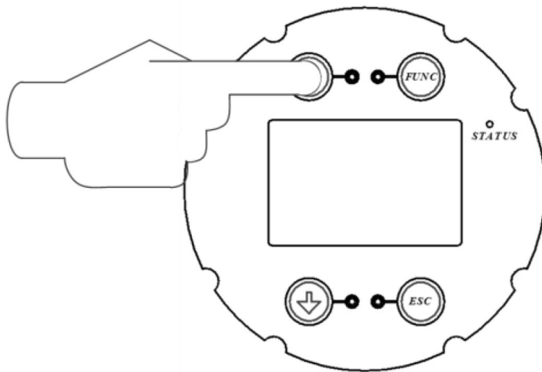
Рисунок 14 - Управление сенсорными клавишами
