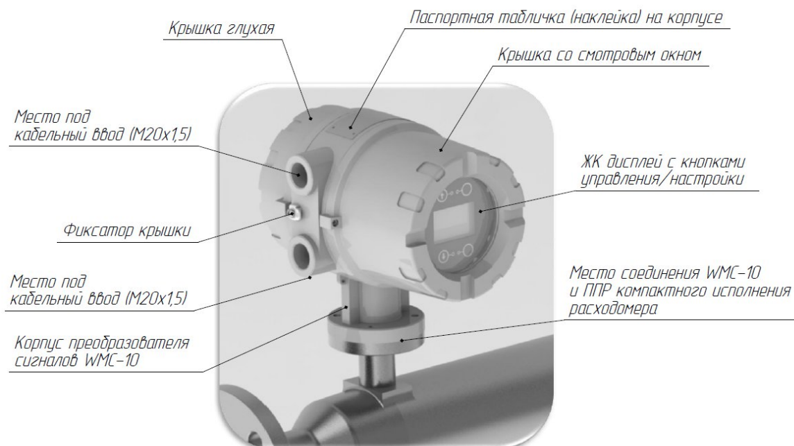
Рисунок 3 – Основные элементы преобразователя сигналов WMC-10I интегрального исполнения расходомера
