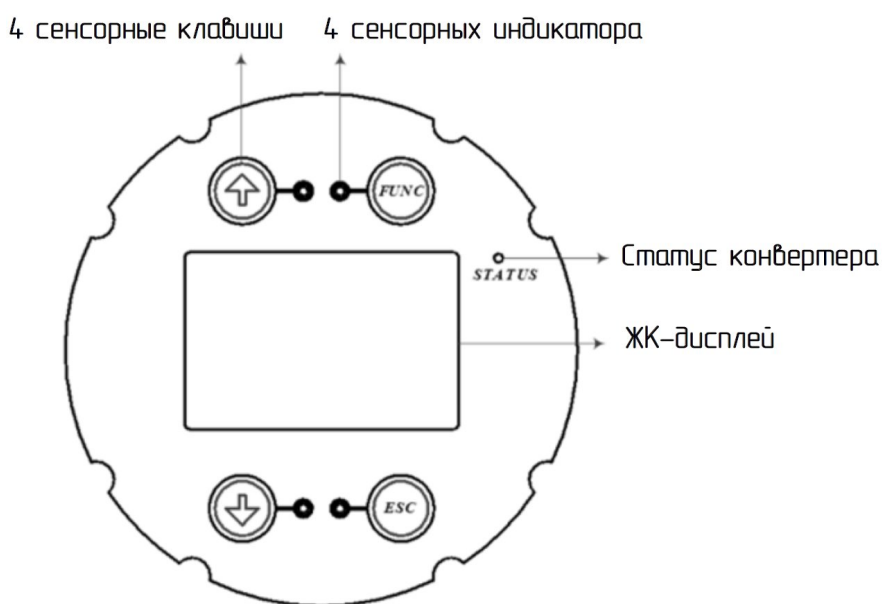
Рисунок 13 - ЖК-дисплей и сенсорная клавиатура
