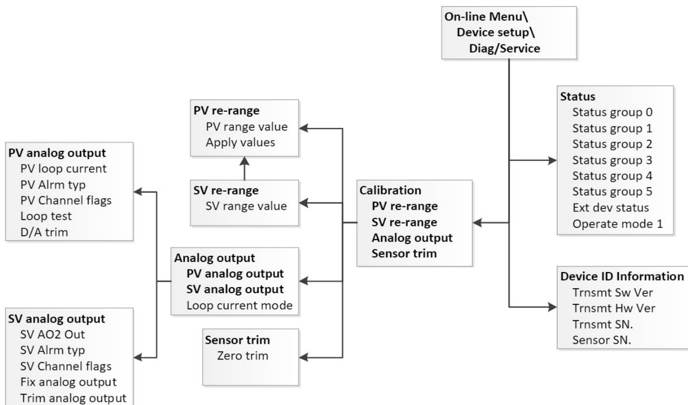
Рисунок 22 – Дерево меню раздела «Diag/Service»
