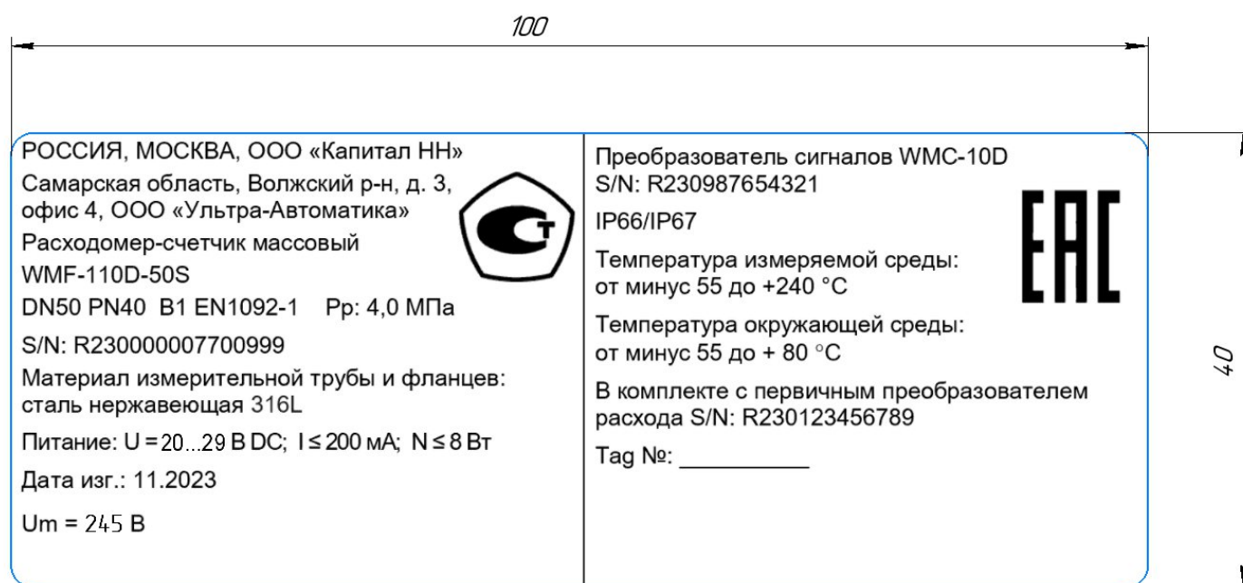
Рисунок 5а – Пример паспортной таблички на корпусе преобразователя сигналов WMC-10
