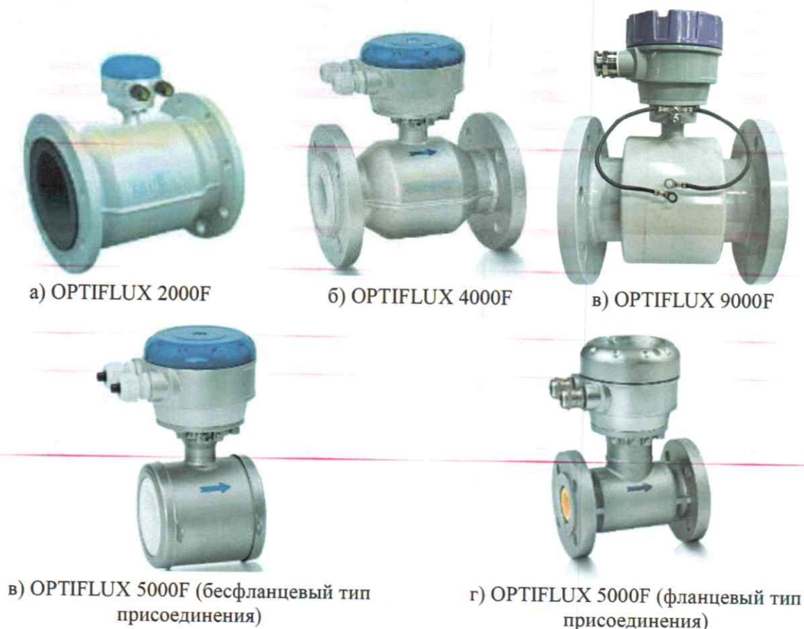
Рисунок 2 – Общий вид первичных преобразователей (раздельное исполнение)
