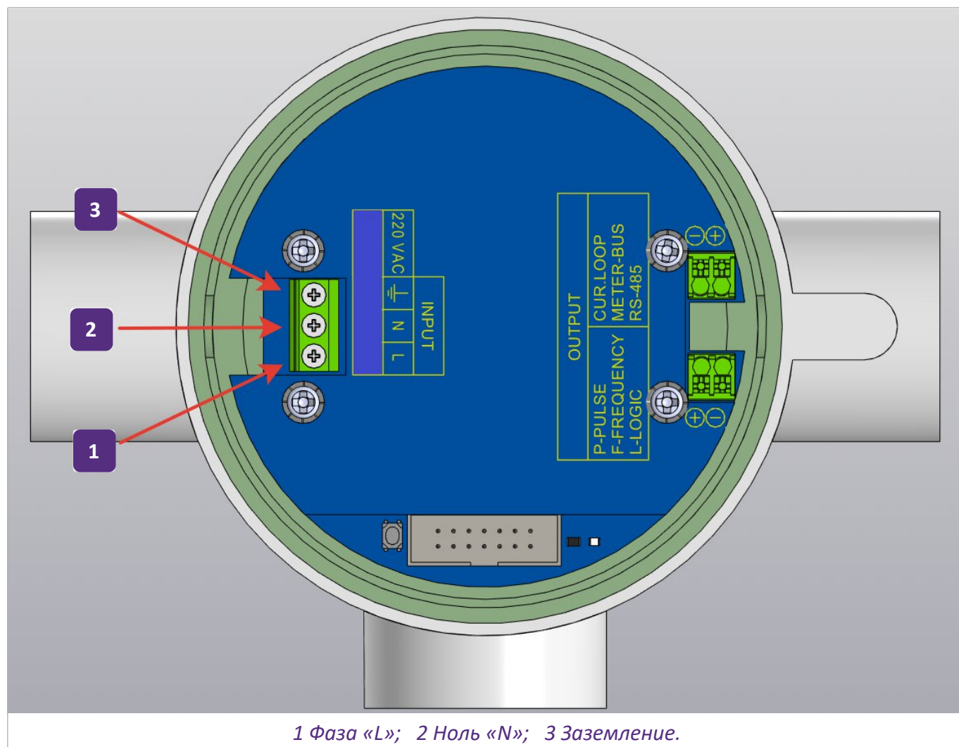
Рисунок 22 – Клеммы для подключения питания 100-230В (-15%/+30%, переменный ток) к ПС
