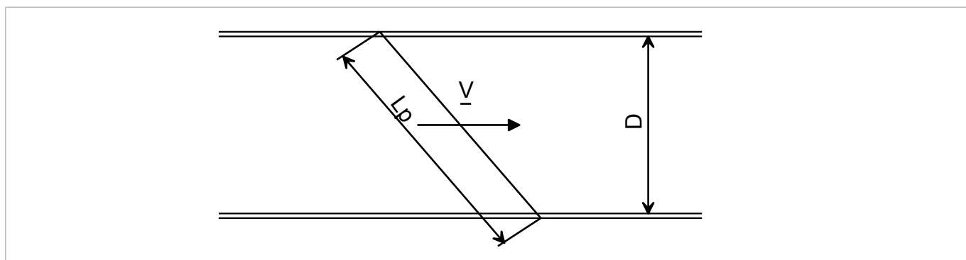
Рисунок 4 — Расположение сенсоров в ПРП
