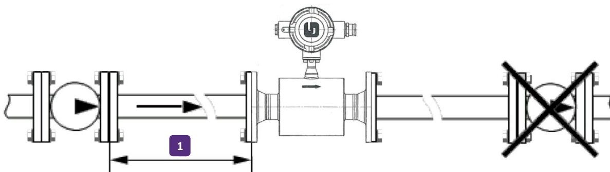
Рисунок 16 – Расположение насоса
