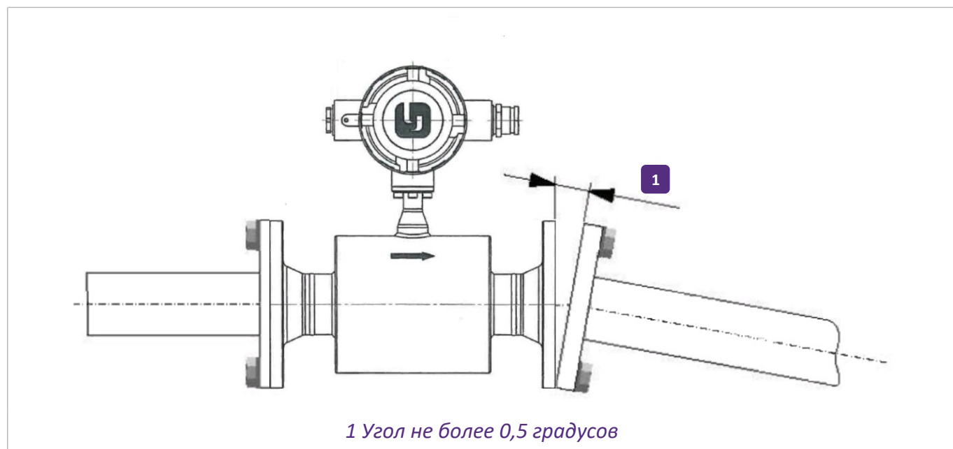
Рисунок 18 – Положение фланцев
