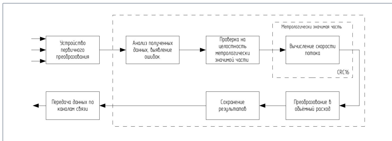
Рисунок 68 – Структурная схема принципа работы измерений
