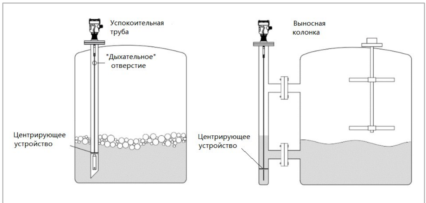
Рисунок 18 – Монтаж в успокоительной или на выносной колонке
