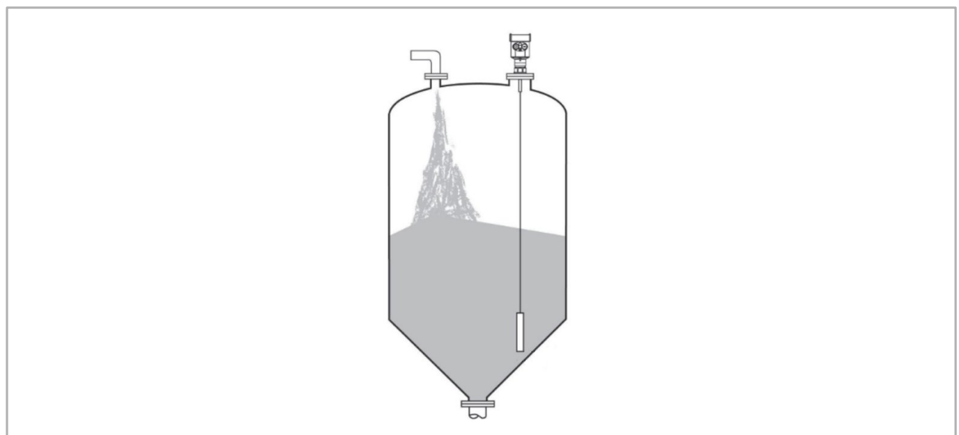
Рисунок 14 – Монтаж уровнемера при наличии устройств загрузки и выгрузки среды
