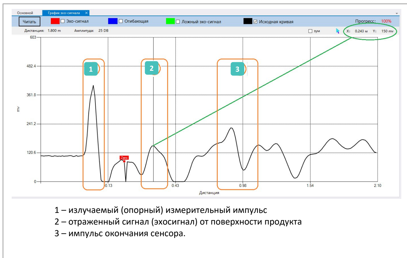
Рисунок А-8 – Исходная эхограмма
