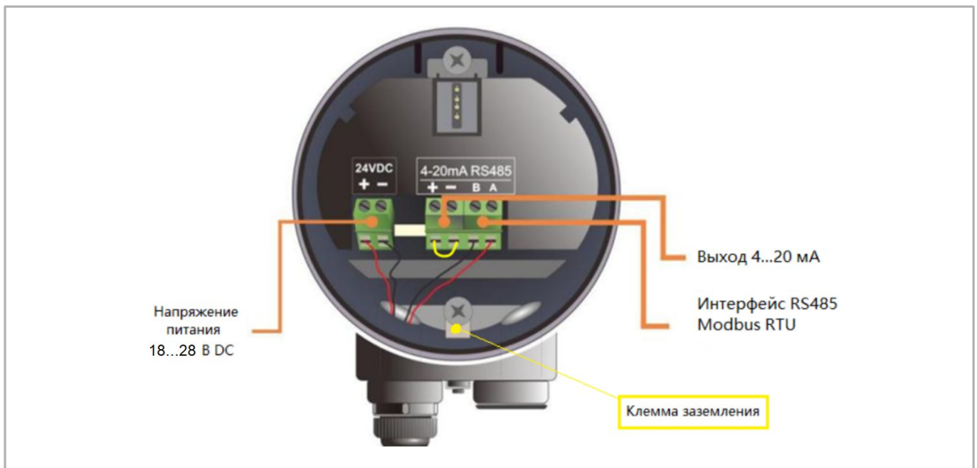
Рисунок 20 – Схема подключения рефлекс-радарного уровнемера с интерфейсом RS485 Modbus RTU
