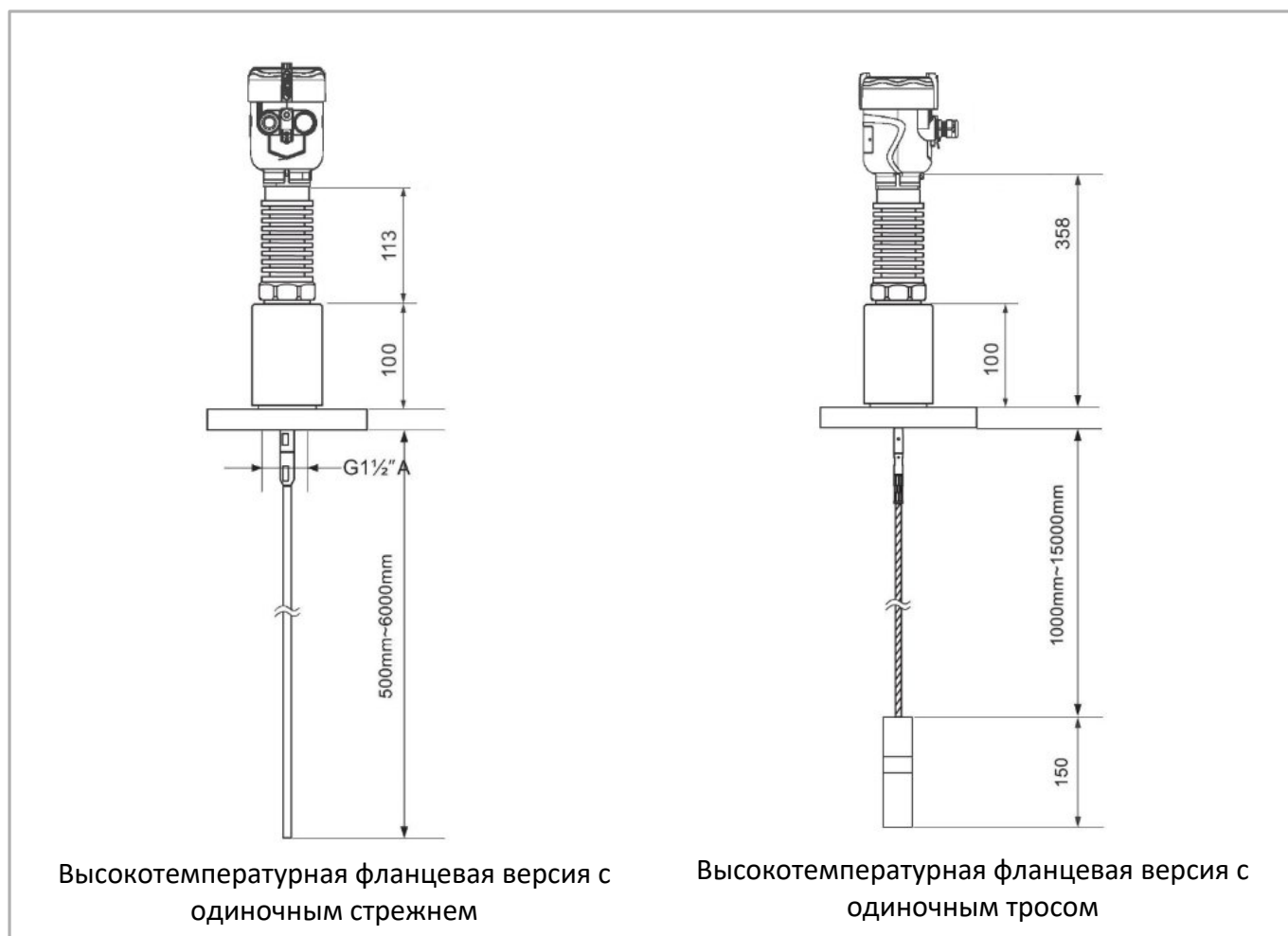
Рисунок 7 – Размеры уровнемеров
