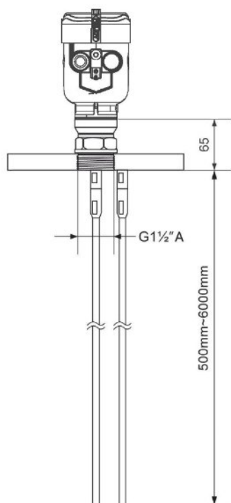
Резьбовая версия с двойным стержнем
